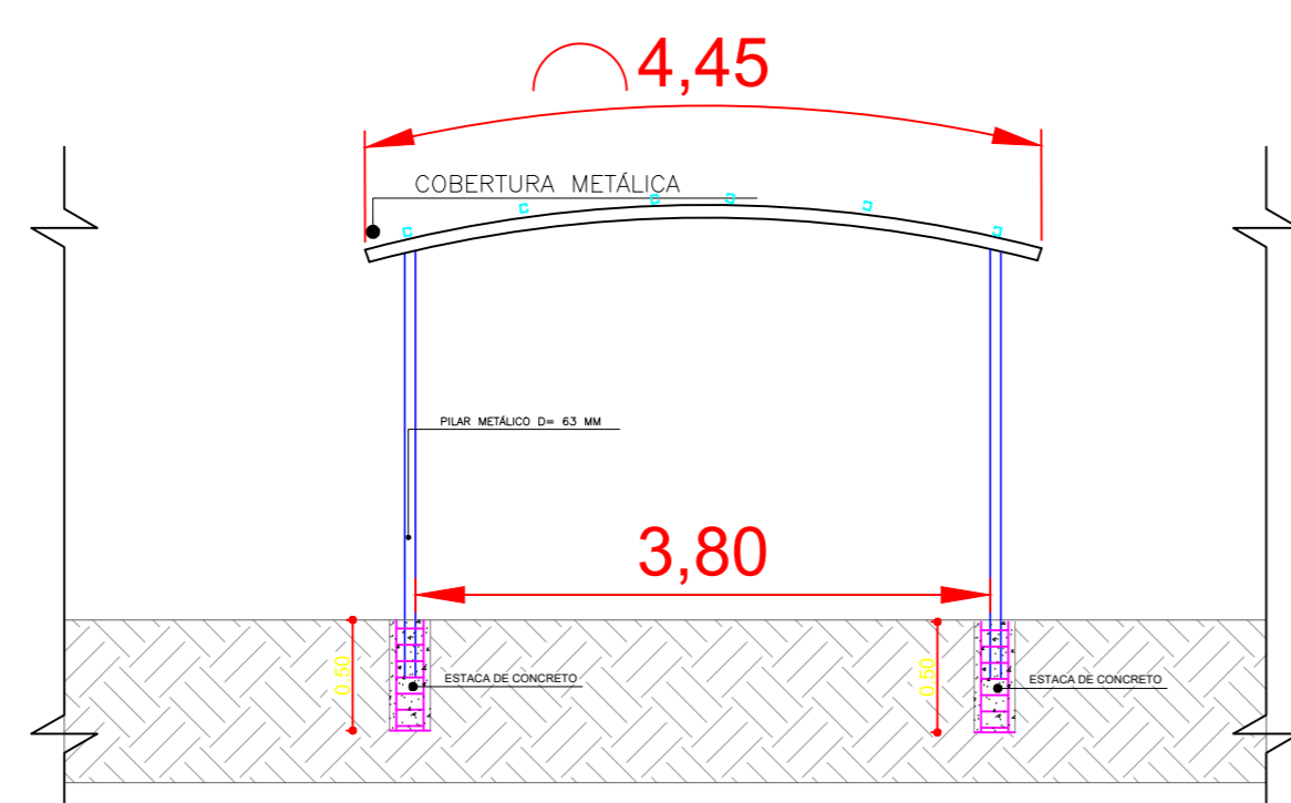
DETALHE 03 - COBERTURA METÁLICA ESC.: 1/50
