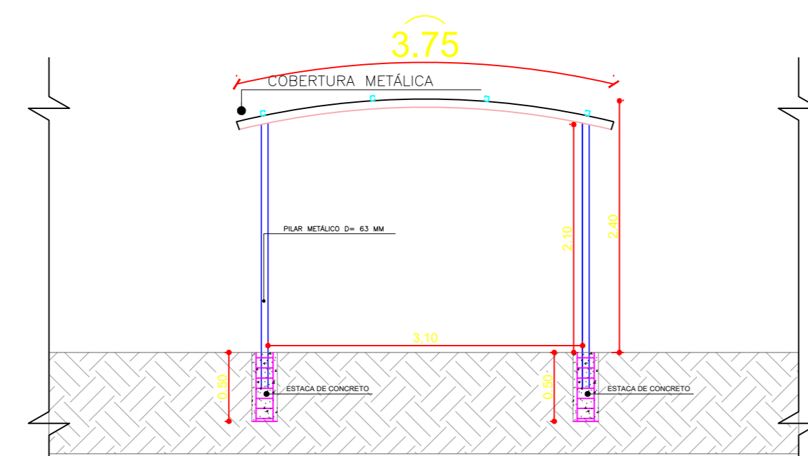
DETALHE 02 - COBERTURA METÁLICA ESC.: 1/50
