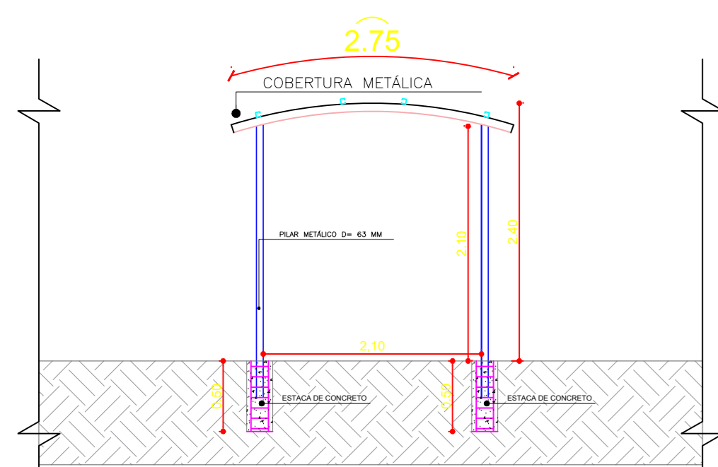
DETALHE 01 - COBERTURA METÁLICA ESC.: 1/50
