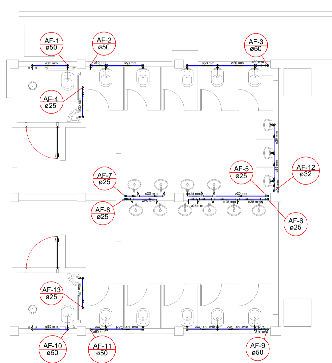
PLANTA BAIXA SANITÁRIO TÉRREO escala 1/50
