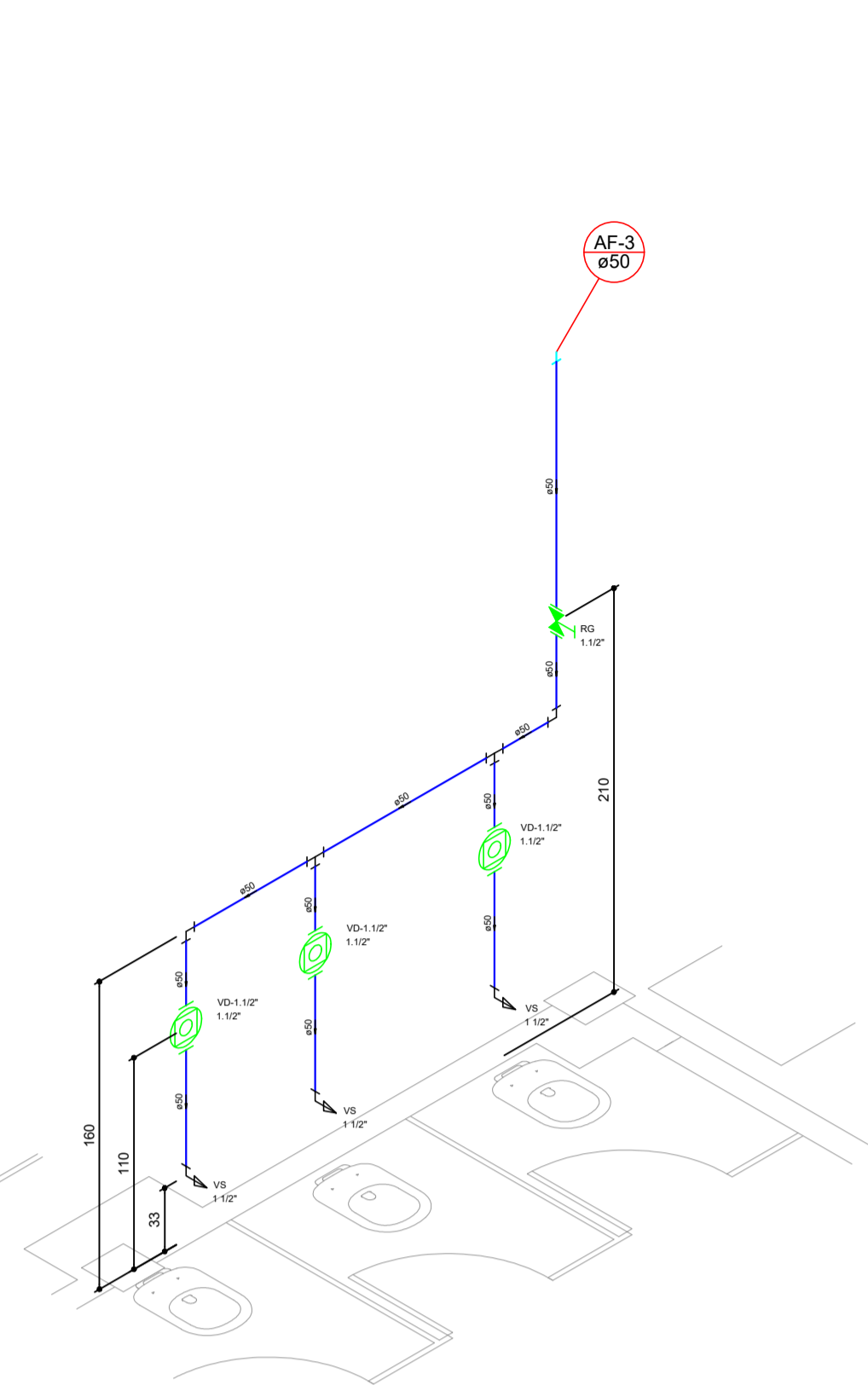
DETALHE 02 escala 1:25
