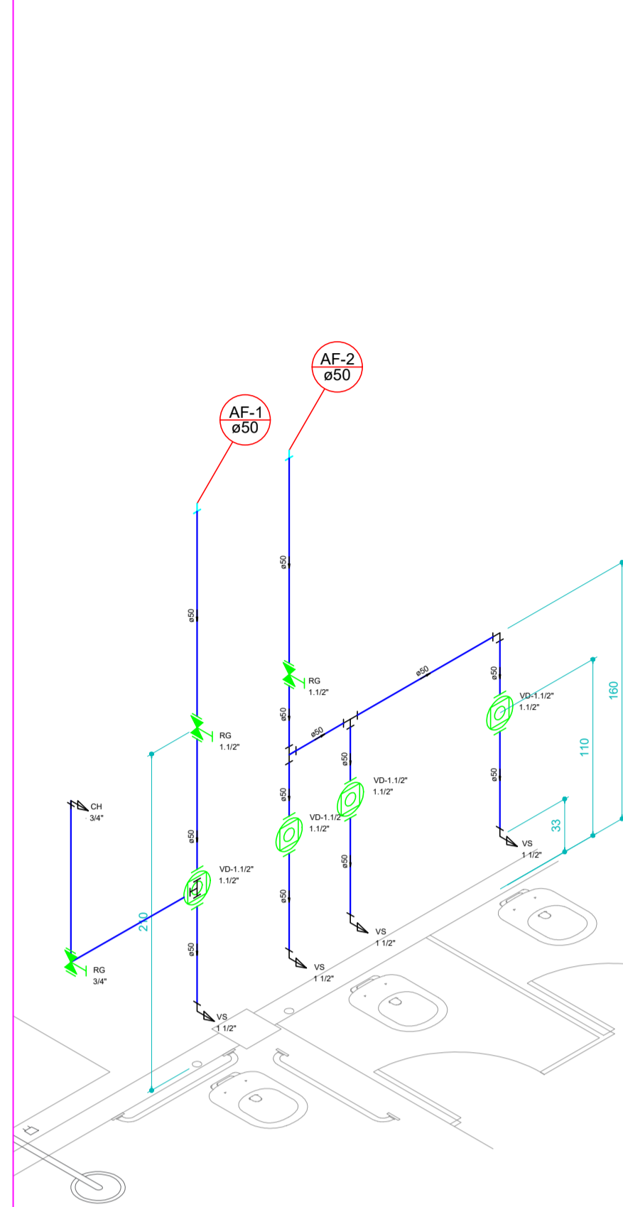
DETALHE 01 escala 1:25
