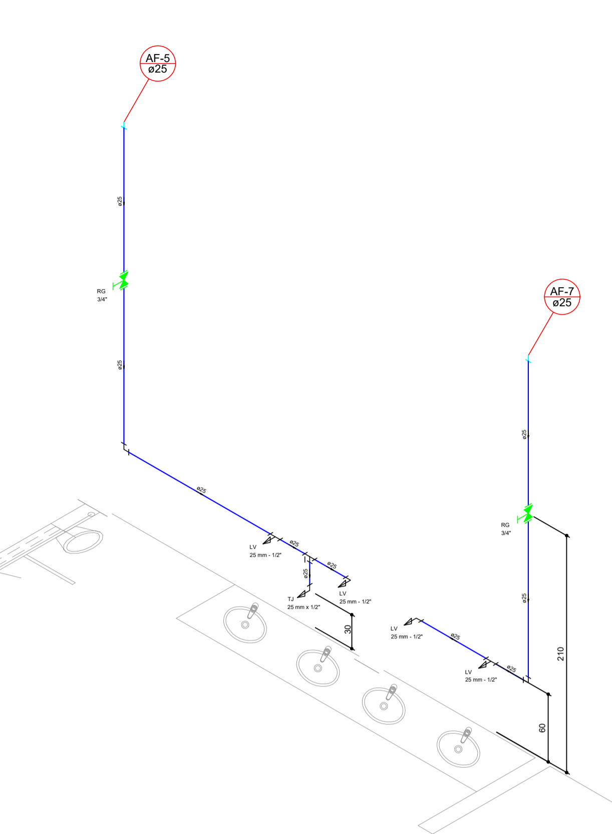
DETALHE 04 escala 1:25
