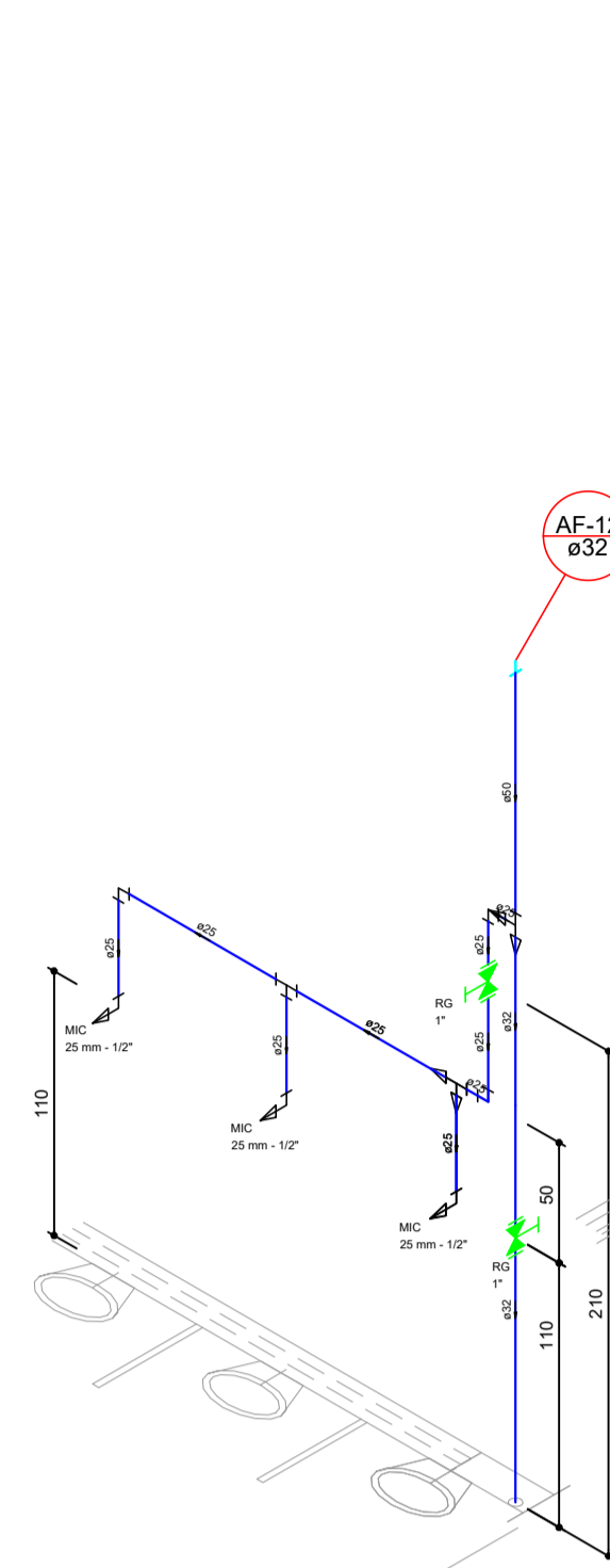
DETALHE 03 escala 1:25
