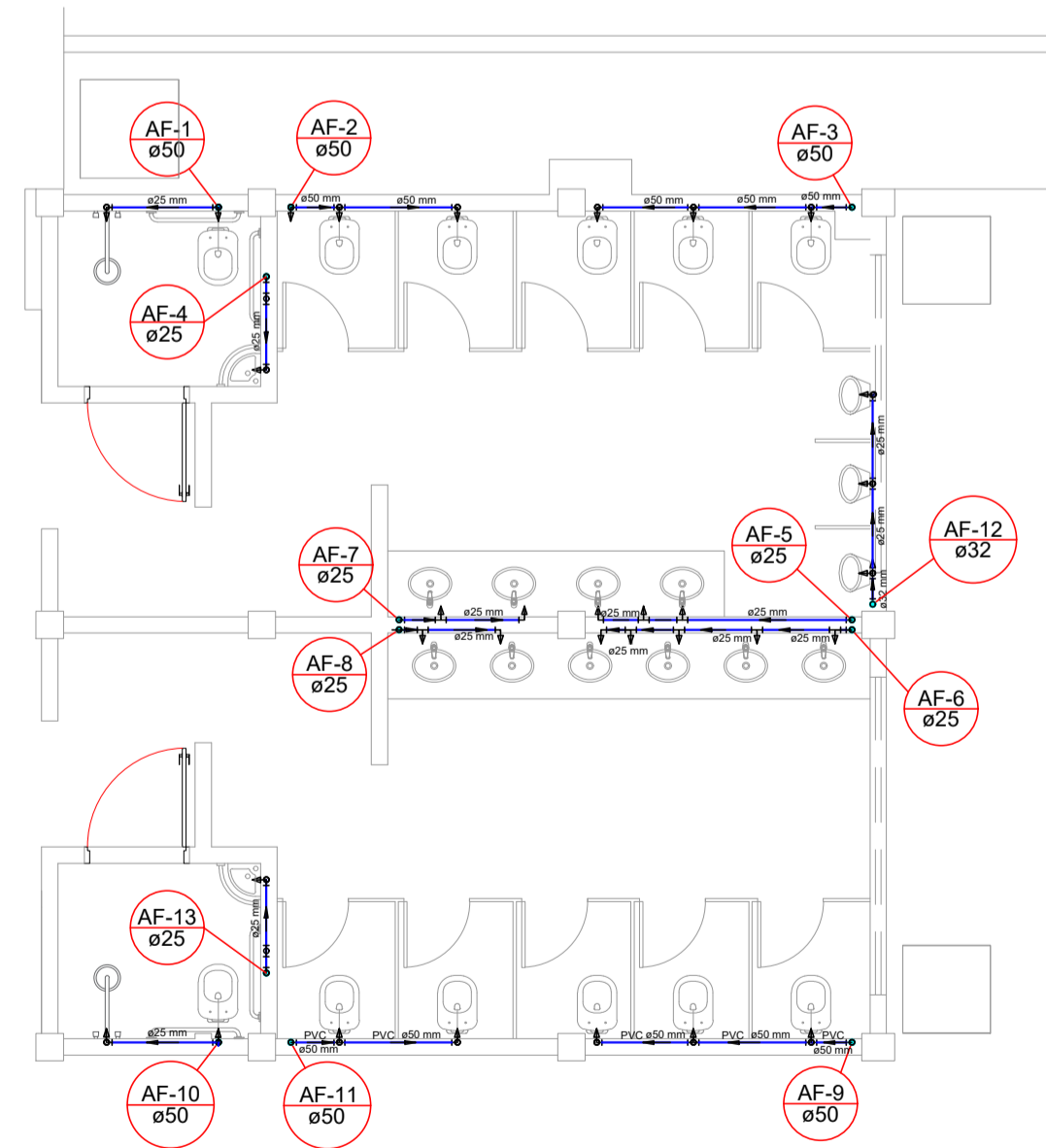
PLANTA BAIXA SANITÁRIO 1º PAV. escala 1/50
