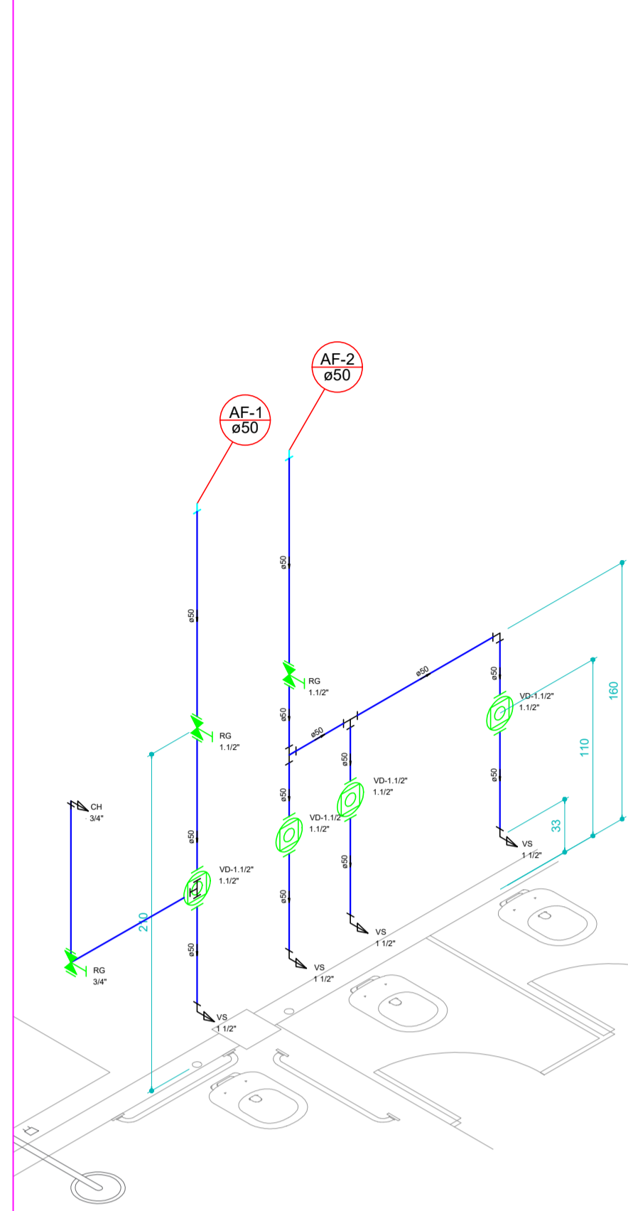
DETALHE 01 escala 1:25
