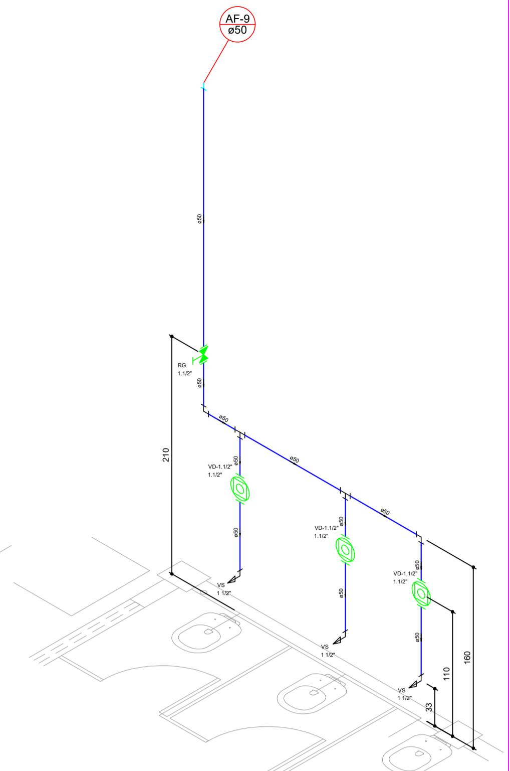
DETALHE 06 escala 1:25
